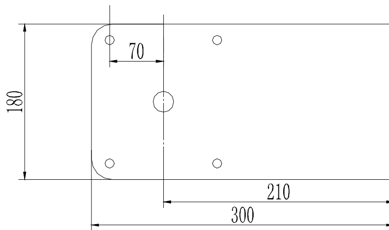
End Elevation
